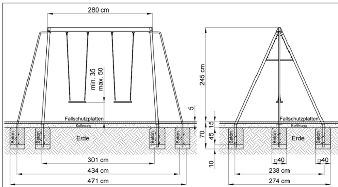
Kinderschaukel MAXI Typ 2K
