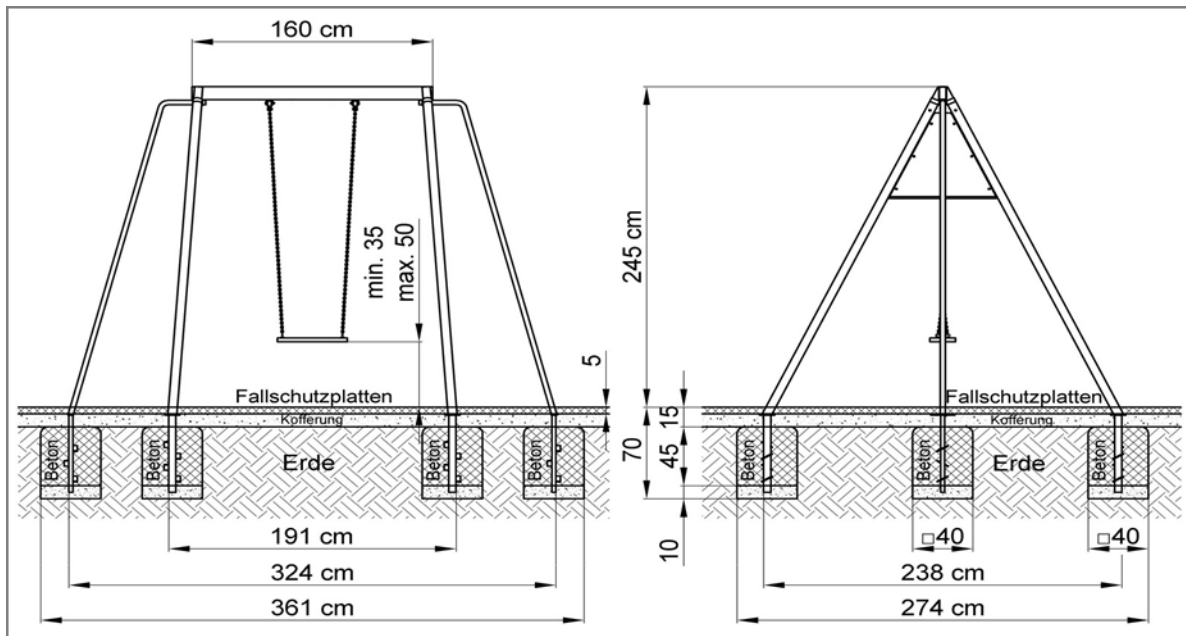
Kinderschaukel MAXI Typ 1K
